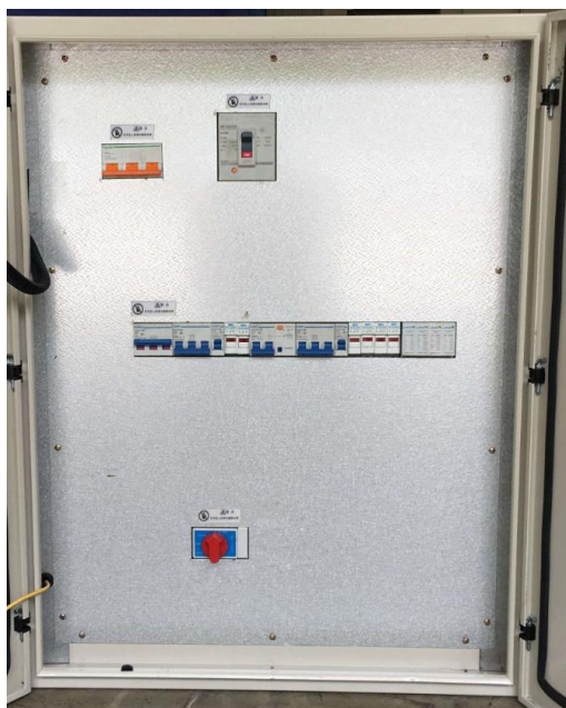
操作面照片
