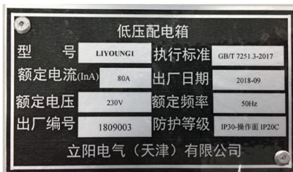
铭牌照片
