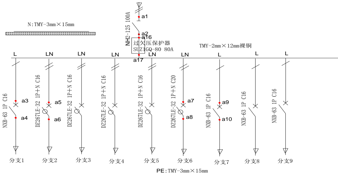
温升示意图 F1:
